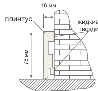
Крепление плинтуса на жидкие гвозди
