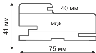
Коробка Телескоп-40(41*75) МДФ Frame Telescope -40(41*75) MDF
