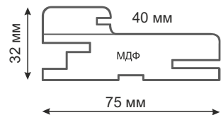
Коробка Телескоп-40(32*75) МДФ Frame Telescope -40(32*75) MDF
