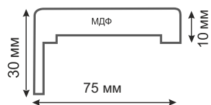
Наличник MR-T (10*75) МДФ Trim MR-T (10*75) MDF
