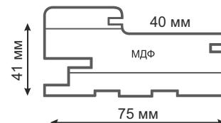
Коробка Компланар 40 (41*75) МДФ Frame Coplanar 40 (41*75) MDF
