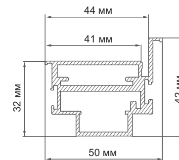
Алюминиевый короб/ Aluminum Box
