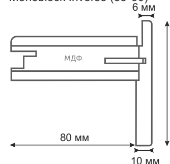
Моноблок Инверсо (85*90) Monoblock Inverso (85*90)
