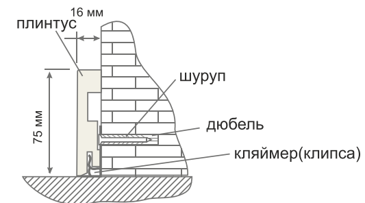
Крепление плинтуса с помощью кляймера (клипсы)
